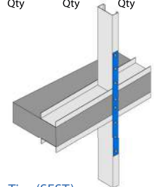
StrapTies (SFST) SFST2-33x2 SFST2-43x2 SFST2-33x4 SFST2x43x2 Qty Qty Qty Qty
