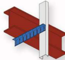
StrutFlex Slide Clip (SFSF) SFSF1200 SFSF1600 SFSF2000 SFSF2400 Qty Qty Qty Qty
